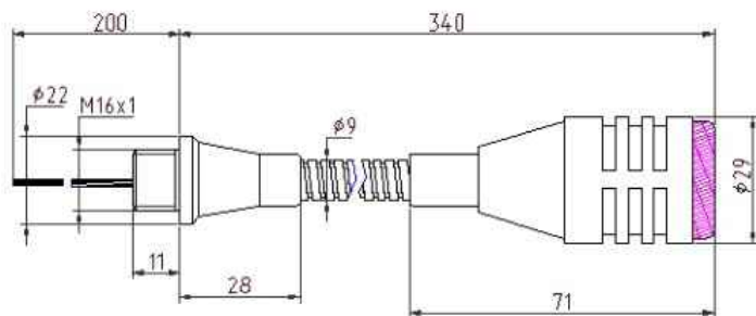
Габаритный чертеж
