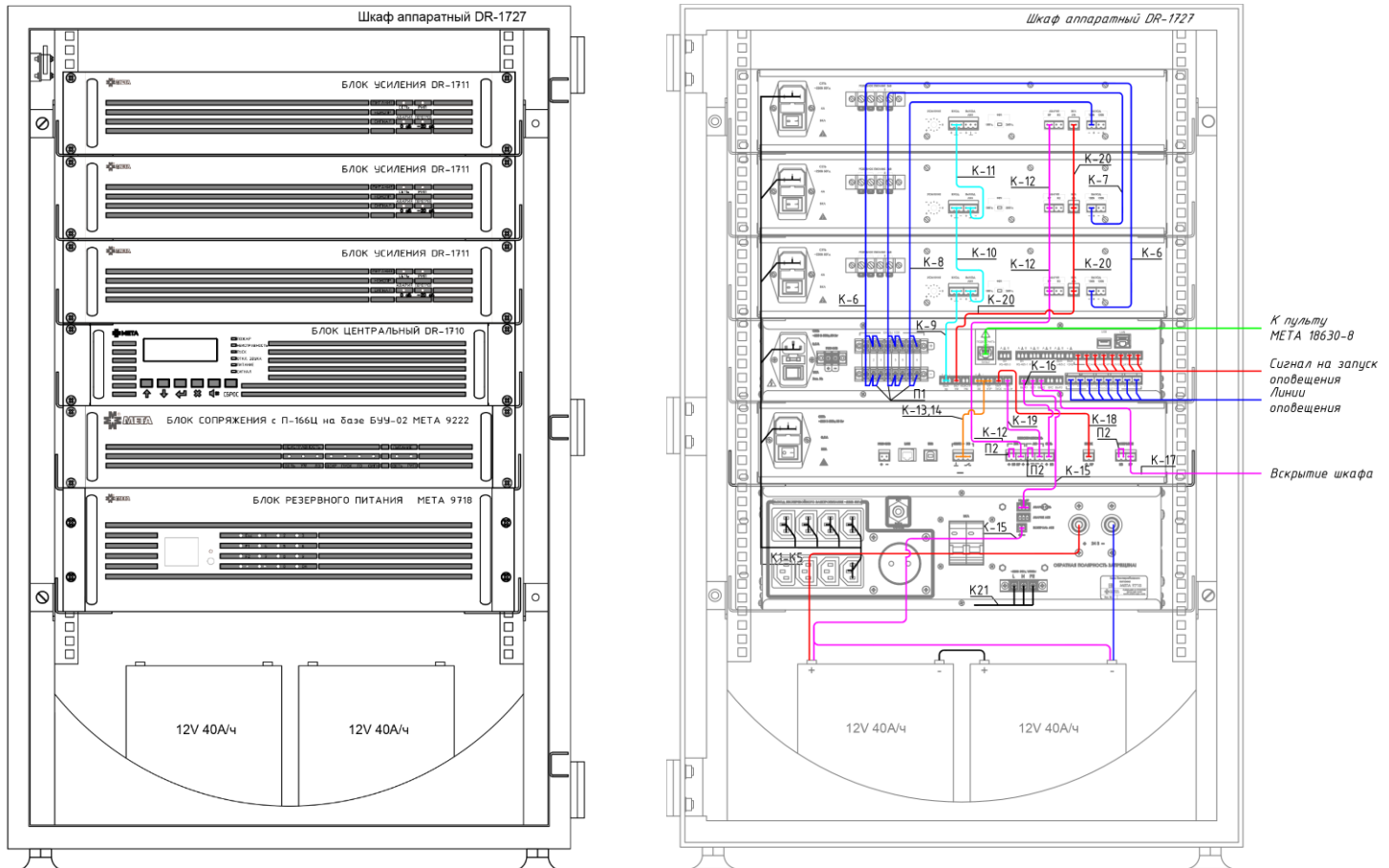
Рисунок 1. Внешний вид УКК МЕТА 8801-09.
