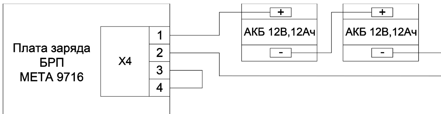
Рисунок 4. Схема подключения АКБ к БРП МЕТА 9716.
