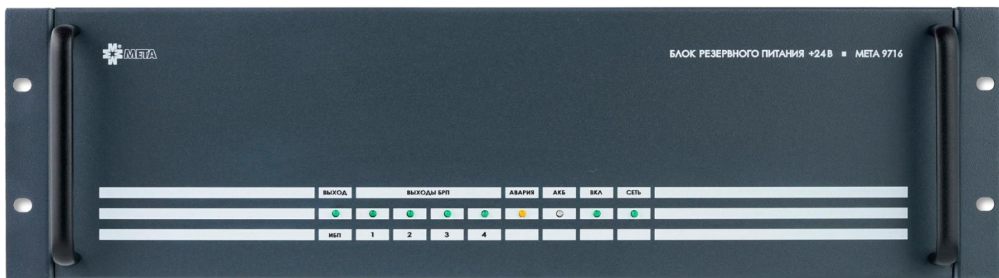
Рисунок 2. Органы индикации БРП МЕТА 9716.
