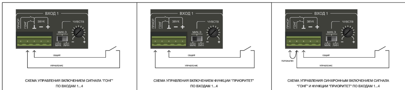
Рисунок 5. Схема подключения устройств управления к входам 1÷4.
