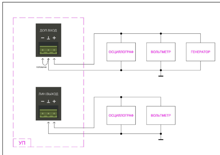
Рисунок 12. Схема измерений по входу «ДОП.ВХОД».
