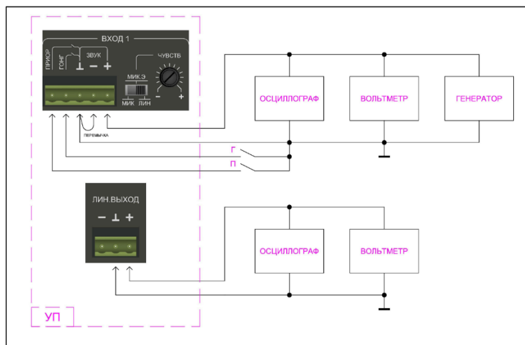
Рисунок 11. Схема измерений по входам «ВХОД 1»...«ВХОД 4».
