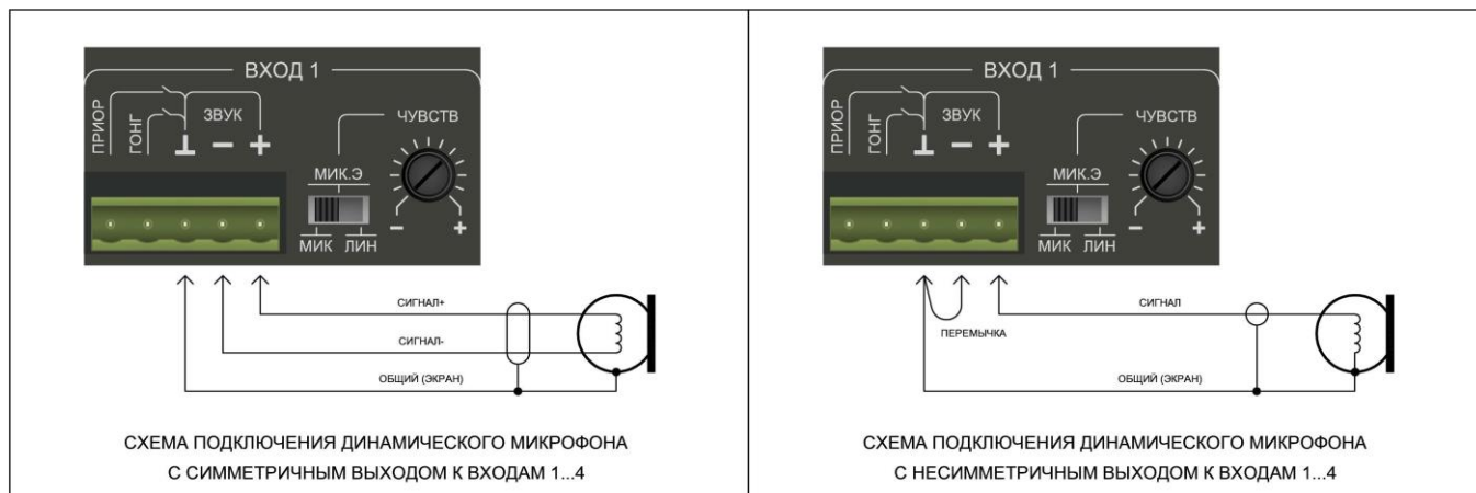
Рисунок 2. Схема подключения динамического микрофона к входам 1÷4.
