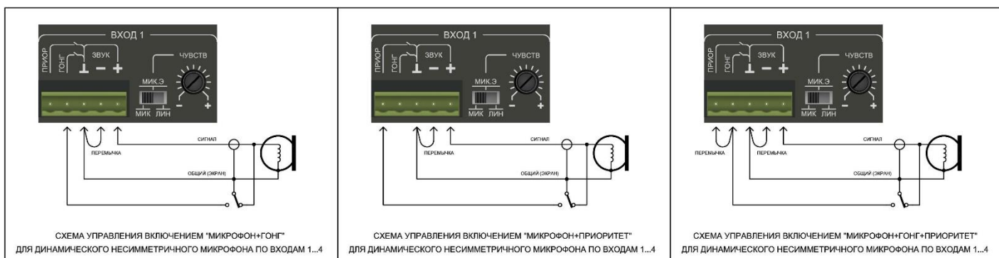
Рисунок 6. Схема подключения динамического микрофона к входам 1÷4.
