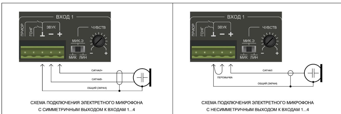
Рисунок 3. Схема подключения электретного микрофона к входам 1÷4.
