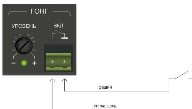
Рисунок 8. Схема подключения устройств управления включением сигнала ГОНГ.
