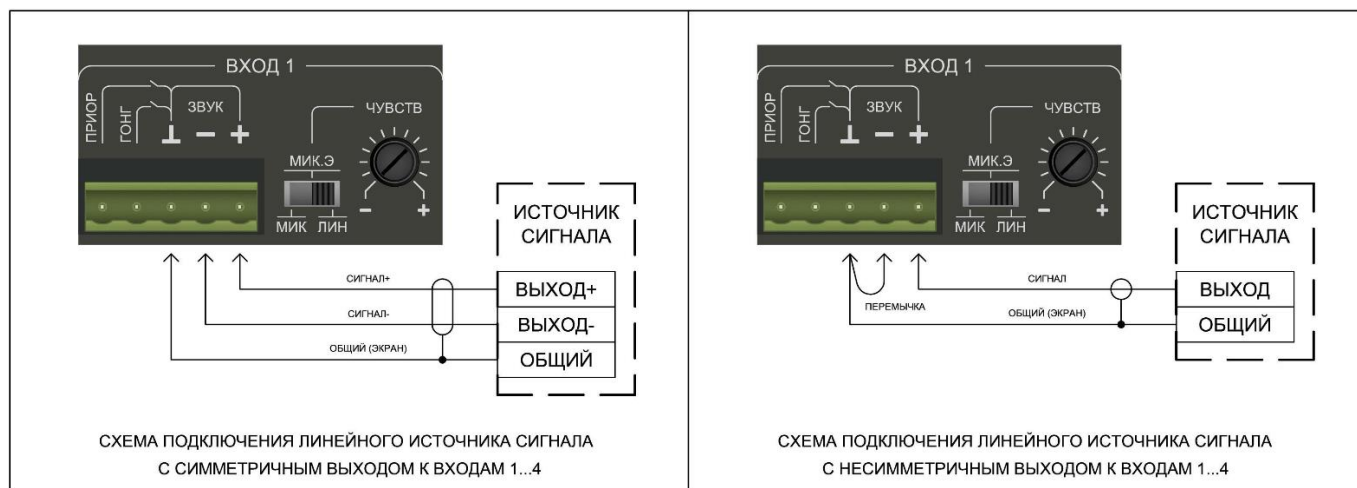
Рисунок 4. Схема подключения источника линейного сигнала к входам 1÷4.
