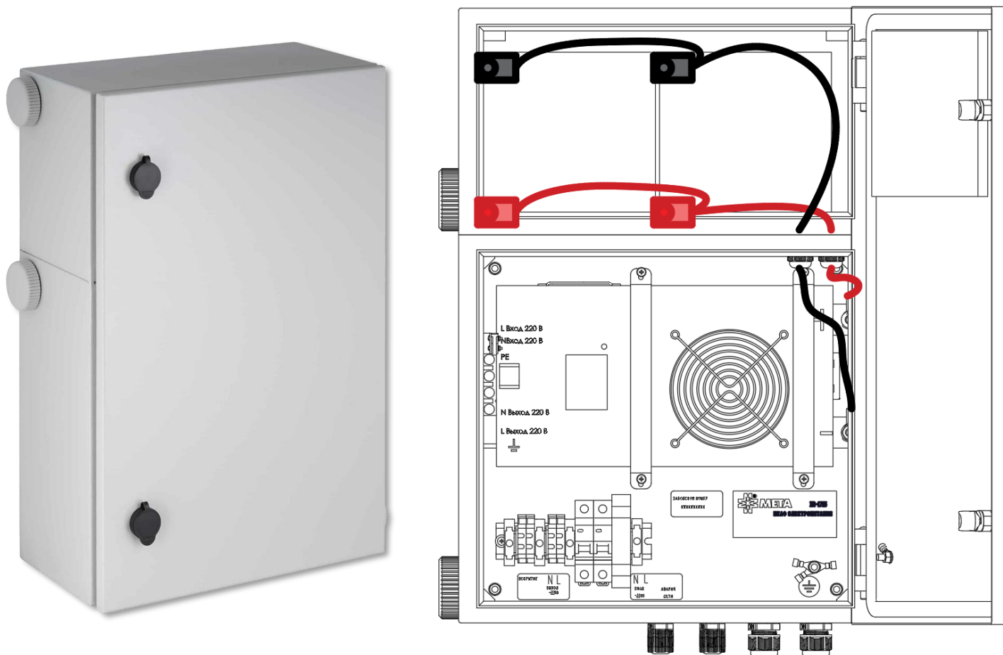
Рисунок 1. Внешний вид ИИЭ DR 1715.
