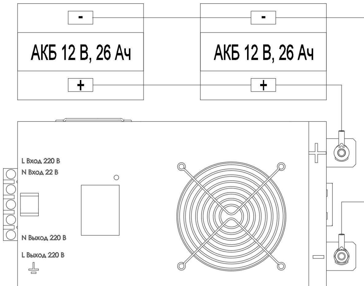
Рисунок 2. Схема подключения АКБ к ШЭ DR 1715.
