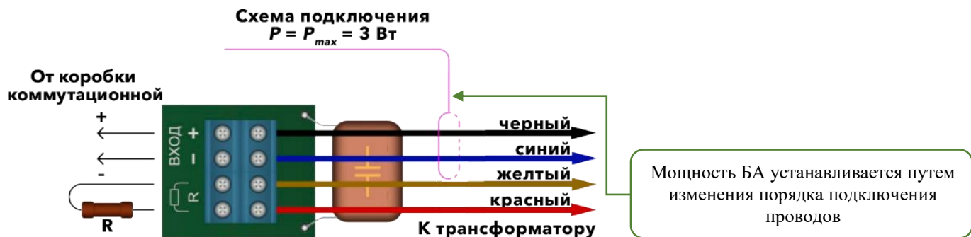
Рисунок 10.1. Схема подключения и установки мощности P_{max} = 3 \text{ Вт} БА АСР-03.1.7 исп. XX.KX с пластиковой клеммной колодкой, с элементом контроля по постоянному току.
