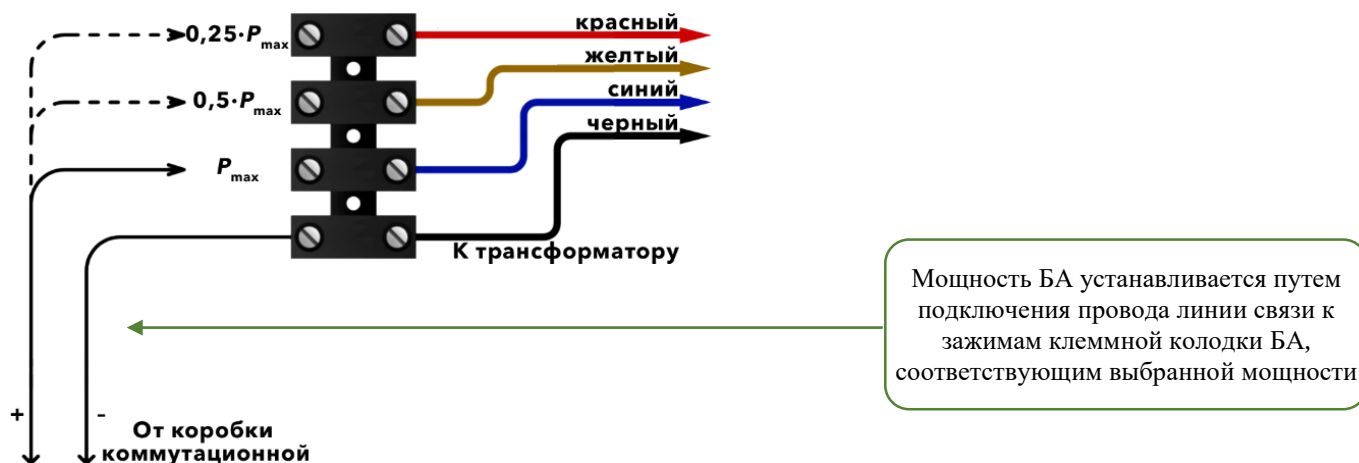
Рисунок 5. Схема подключения и установки мощности БА АСР-03.1.7 исп. XX.AX с полиэтиленовой клеммной колодкой, с возможностью контроля по переменному току (импедансу).
