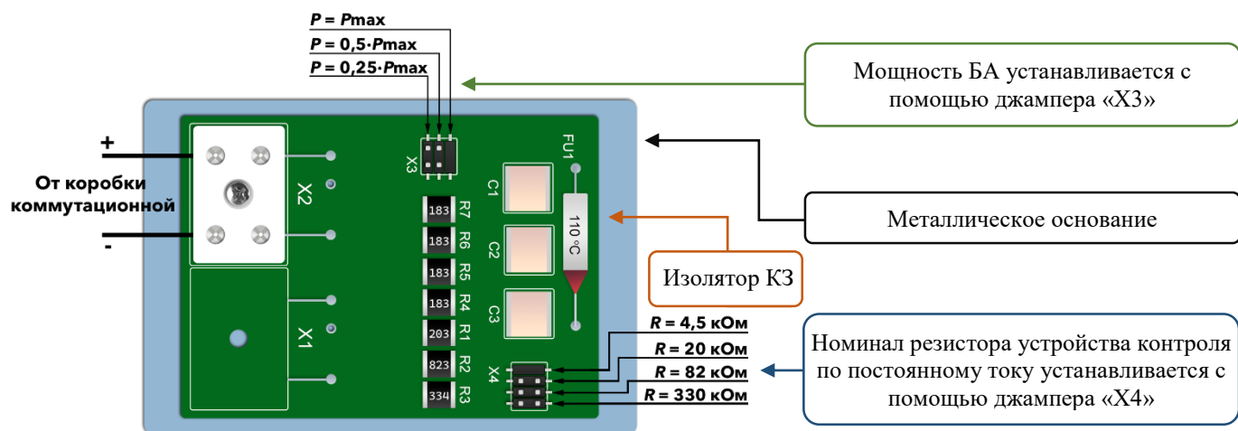
Рисунок 9. Схема подключения и установки мощности БА АСР-03.1.7 исп. XX.NX с одной керамической клеммной колодкой на металлическом основании, с изолятором КЗ, с устройством контроля по постоянному току.
