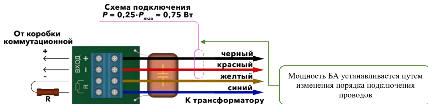
Рисунок 10.3. Схема подключения и установки мощности 0,25 \cdot P_{\max} = 0,75 \text{ Вт} БА АСР-03.1.7 исп. XX.KX с пластиковой клеммной колодкой, с элементом контроля по постоянному току.
