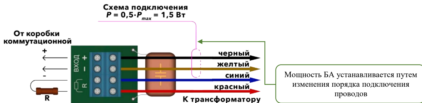
Рисунок 10.2. Схема подключения и установки мощности 0,5 \cdot P_{\max} = 1,5 \text{ Вт} БА АСР-03.1.7 исп. XX.KX с пластиковой клеммной колодкой, с элементом контроля по постоянному току.
