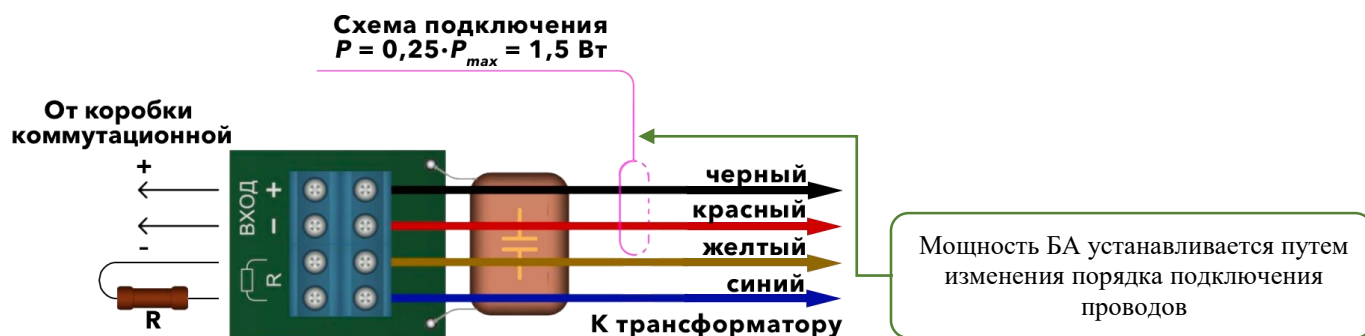
Рисунок 10.3. Схема подключения и установки мощности 0,25 \cdot P_{\max} = 0,75 \text{ Вт} БА АСР-06.1.7 исп. XX.KX с пластиковой клеммной колодкой, с элементом контроля по постоянному току.
