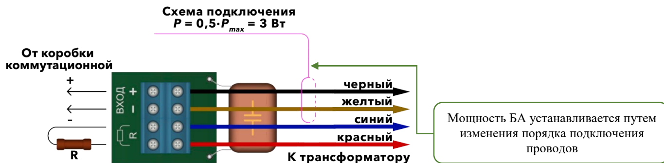
Рисунок 10.2. Схема подключения и установки мощности 0,5 \cdot P_{\max} = 1,5 \text{ Вт} БА АСР-06.1.7 исп. XX.KX с пластиковой клеммной колодкой, с элементом контроля по постоянному току.
