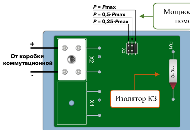
Рисунок 6. Схема подключения и установки мощности БА АСП-06.1.7 исп. XX.BX с одной керамической клеммной колодкой на металлическом основании, с изолятором КЗ, с возможностью контроля по переменному току (импедансу).
