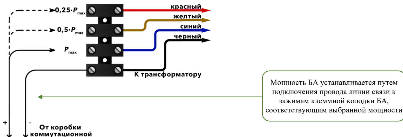
Рисунок 5. Схема подключения и установки мощности БА АСП-06.1.7 исп. XX.AX с полиэтиленовой клеммной колодкой, с возможностью контроля по переменному току (импедансу).
