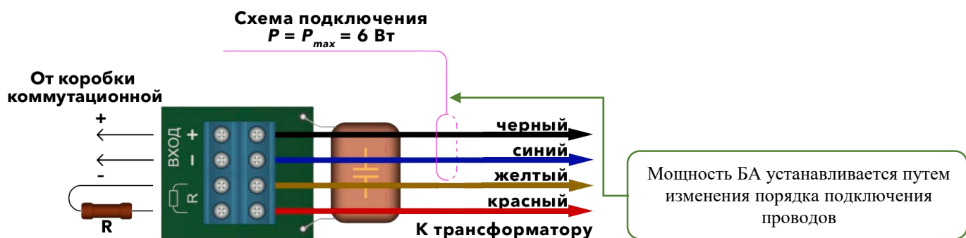
Рисунок 10.1. Схема подключения и установки мощности P_{max} = 3 \text{ Вт} БА АСР-06.1.7 исп. XX.KX с пластиковой клеммной колодкой, с элементом контроля по постоянному току.
