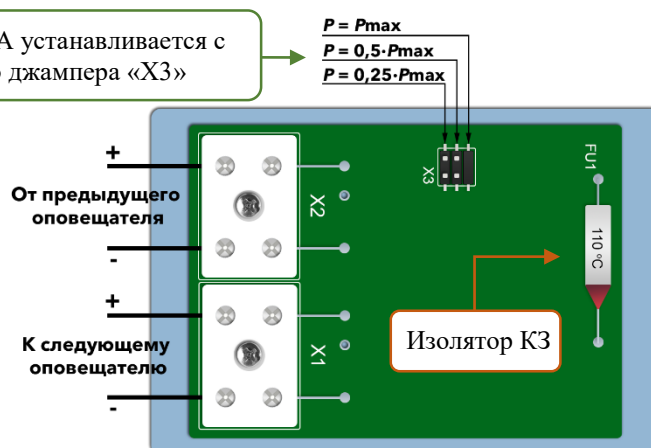
Рисунок 7. Схема подключения и установки мощности БА АСП-06.1.7 исп. XX.EX с двумя керамическими клеммными колодками на металлическом основании, с изолятором КЗ, с возможностью контроля по переменному току (импедансу).
