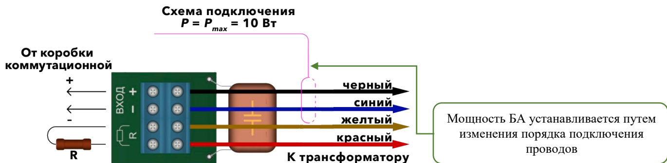
Рисунок 10.1. Схема подключения и установки мощности P_{max} = 10 \text{ Вт} БА АСР-10.1.7 исп. XX.KX с пластиковой клеммной колодкой, с элементом контроля по постоянному току.
