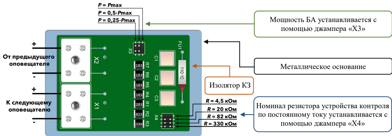
Рисунок 8. Схема подключения и установки мощности БА АСР-10.1.7 исп. XX.MX с двумя керамическими клеммными колодками на металлическом основании, с изолятором К3, с устройством контроля по постоянному току.
