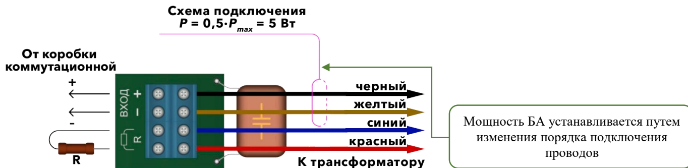
Рисунок 10.2. Схема подключения и установки мощности 0,5 \cdot P_{\max} = 5 \text{ Вт} БА АСР-10.1.7 исп. XX.KX с пластиковой клеммной колодкой, с элементом контроля по постоянному току.
