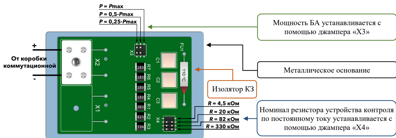
Рисунок 9. Схема подключения и установки мощности БА АСР-10.1.7 исп. XX.NX с одной керамической клеммной колодкой на металлическом основании, с изолятором К3, с устройством контроля по постоянному току.
