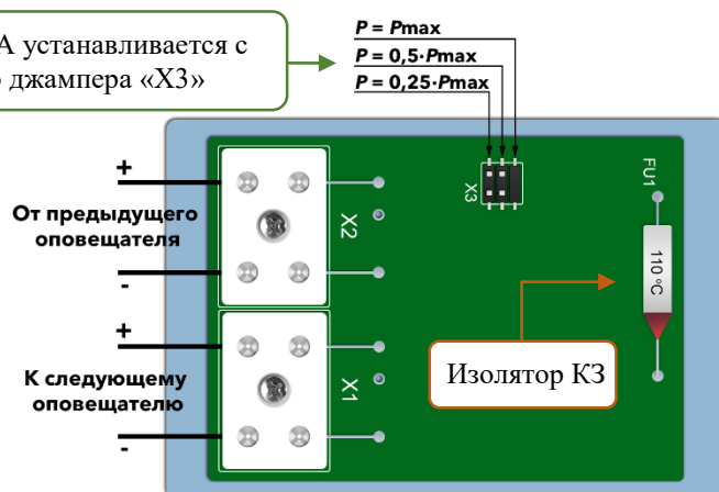
Рисунок 7. Схема подключения и установки мощности БА АСП-10.1.7 исп. XX.EX с двумя керамическими клеммными колодками на металлическом основании, с изолятором КЗ, с возможностью контроля по переменному току (импедансу).
