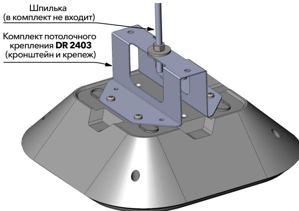
Рисунок 4. Крепление БА АСР-10.1.7 исп. XX.XX к потолку при помощи комплекта потолочного крепления DR 2403.
