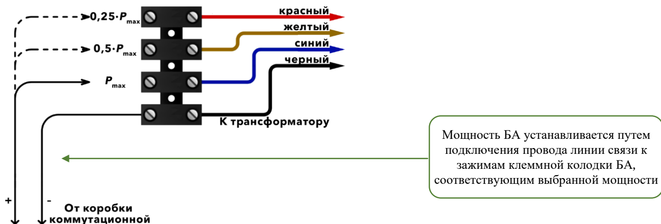
Рисунок 5. Схема подключения и установки мощности БА АСП-10.1.7 исп. XX.AX с полиэтиленовой клеммной колодкой, с возможностью контроля по переменному току (импедансу).
