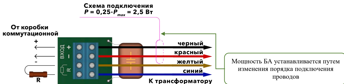
Рисунок 10.3. Схема подключения и установки мощности 0,25 \cdot P_{\max} = 2,5 \text{ Вт} БА АСР-10.1.7 исп. XX.KX с пластиковой клеммной колодкой, с элементом контроля по постоянному току.
