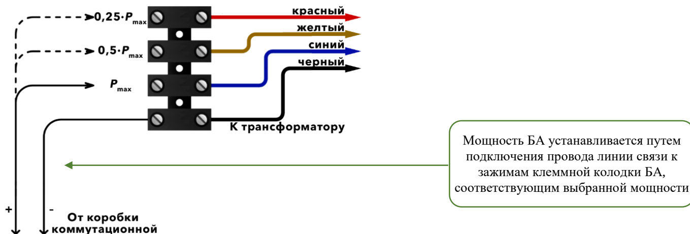
Рисунок 2. Схема подключения и установки мощности БА АСР-01.1.8 исп. XX.АА с полиэтиленовой клеммной колодкой, с возможностью контроля по переменному току (импедансу).
