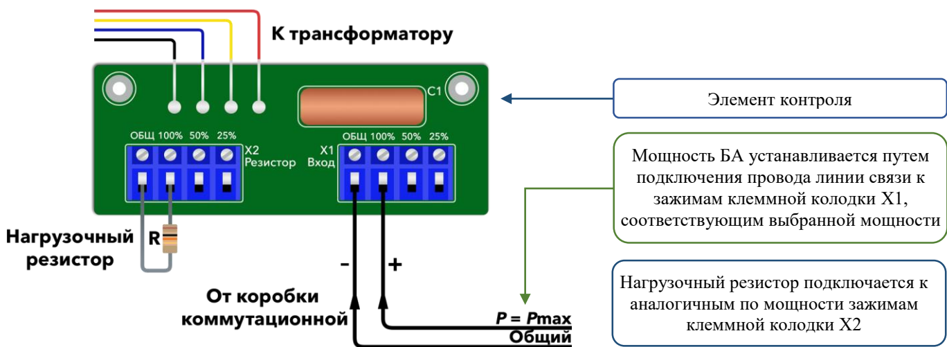
Рисунок 6.1. Схема подключения и установки мощности P_{max} = 1 Вт БА АСР-01.1.8 исп. XX.КА с пластиковыми клеммными колодками, с элементом контроля по постоянному току.
