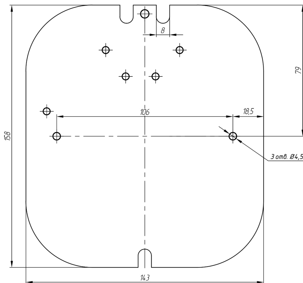
Рисунок 7. Габаритные размеры металлического основания блоков акустических АСР-01.1.8 исп. XX.ЕА, исп. XX.МА и исп. XX.НА.
