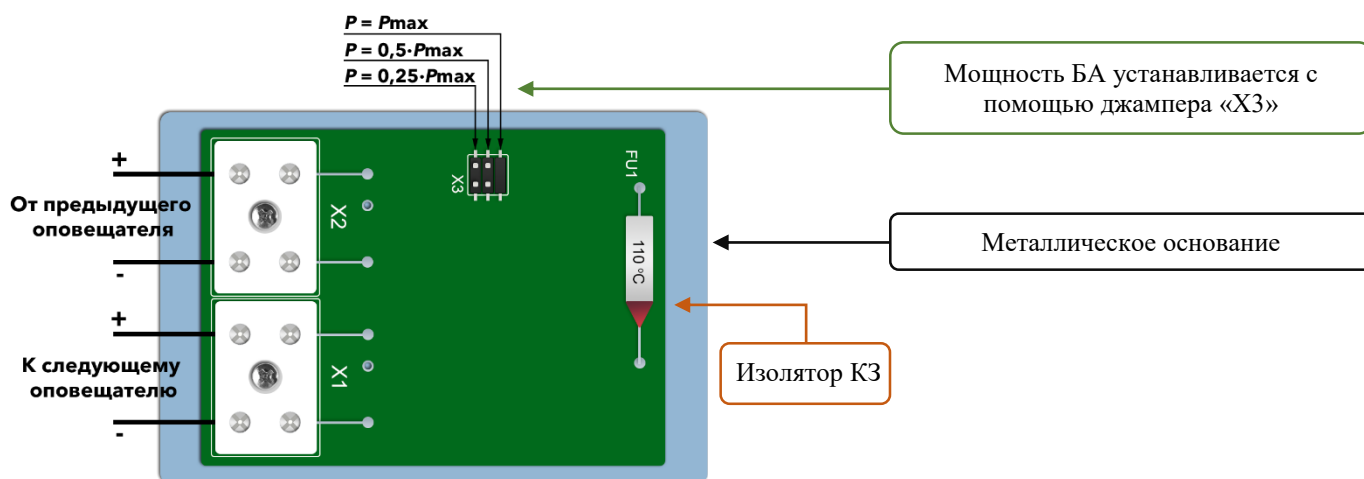
Рисунок 3. Схема подключения и установки мощности БА АСР-03.1.8 исп. XX.ЕА с двумя керамическими клеммными колодками на металлическом основании, с изолятором К3, с возможностью контроля по переменному току (импедансу).
