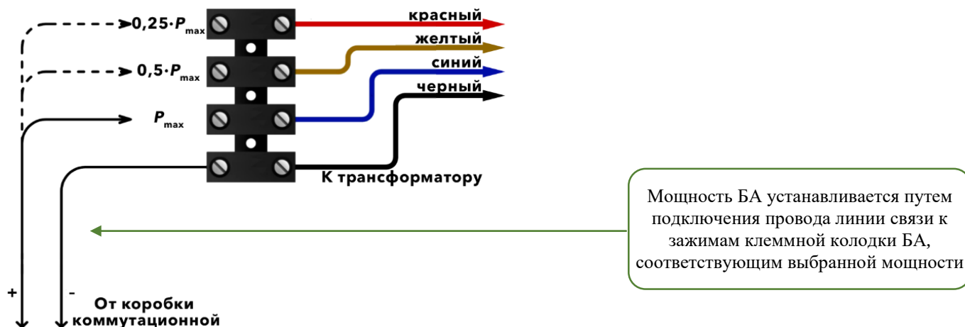
Рисунок 2. Схема подключения и установки мощности БА АСР-03.1.8 исп. XX.АА с полиэтиленовой клеммной колодкой, с возможностью контроля по переменному току (импедансу).
