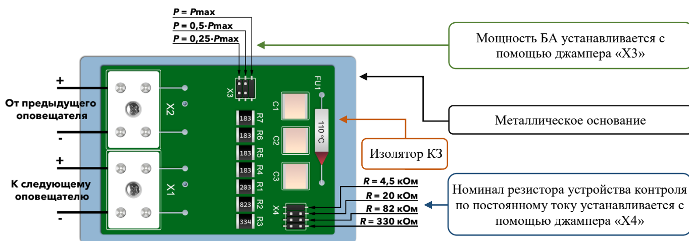
Рисунок 4. Схема подключения и установки мощности БА АСР-03.1.8 исп. XX.МА с двумя керамическими клеммными колодками на металлическом основании, с изолятором К3, с устройством контроля по постоянному току.
