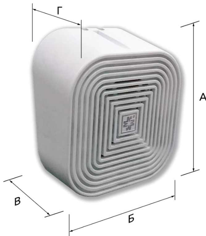
Рисунок 8. Габаритные и установочные размеры блоков акустических АСР-03.1.8 исп. XX.XA.
