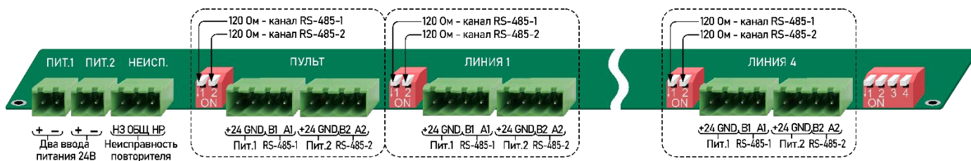
Рисунок 3. Элементы коммутации и управления (терминаторы, клеммы и разъемы) ПИ META 17070/19070.
